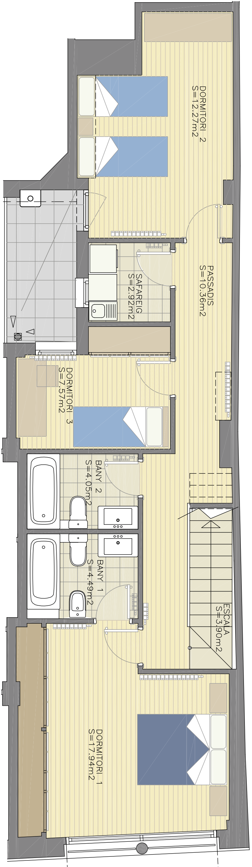
PLANTA CINQUENA (porta 1ª)
